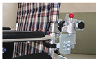
車いす固定スライドブロック (アタッチメントFG19装着時)
