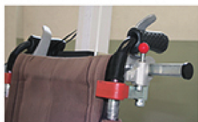
車いす固定スライドブロック(標準時)
